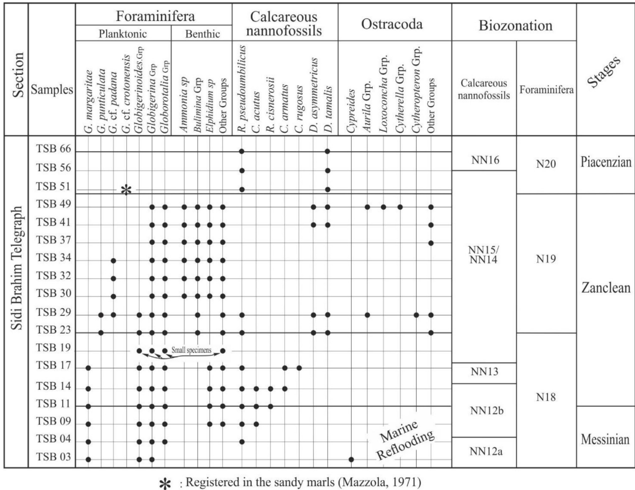
Fig. 9. Stratigraphic distribution of ostracoda, planktonic foraminifera and calcareous nannofossils from the Sidi Brahim Telegraph section Fig. 9. Répartition stratigraphique des ostracodes, des foraminifères planctoniques et des nannofossiles calcaires dans la coupe du Télégraphe de Sidi Brahim.
